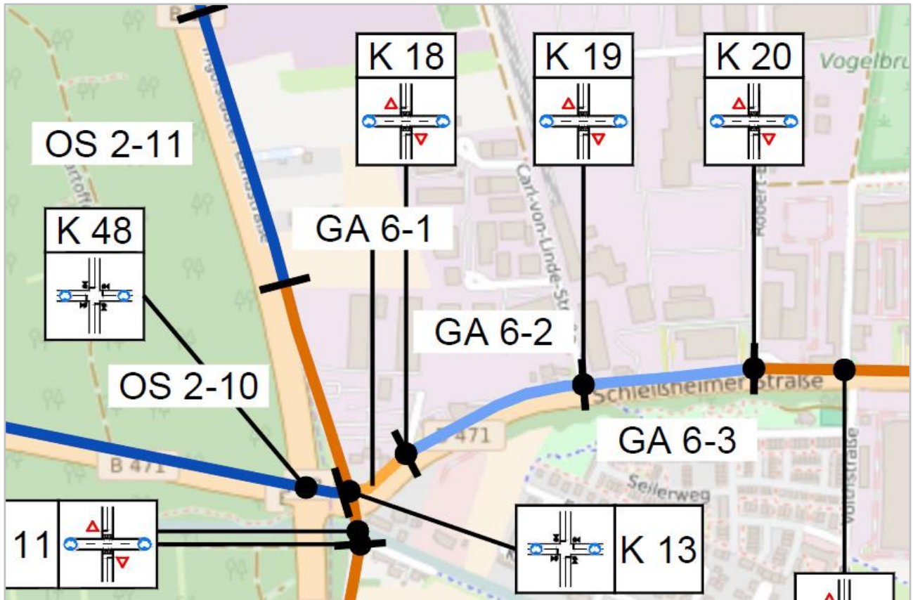
Abb. 35: Streckenabschnitt 9 – Schleißheimer Straße (TÜV Süd bis Robert-Bosch-Straße)
