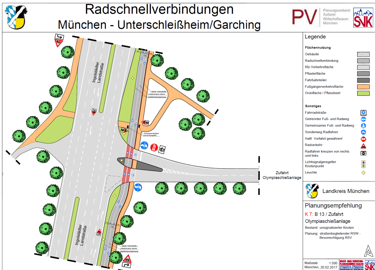
Abb.: Beispielhafte Knotenpunktlösung – Bevorrechtigung eines straßenbegleitenden Radschnellweges an einem vorfahrtgeregeltem Knoten (B 13 / Zufahrt Olympiaschießanlage)
